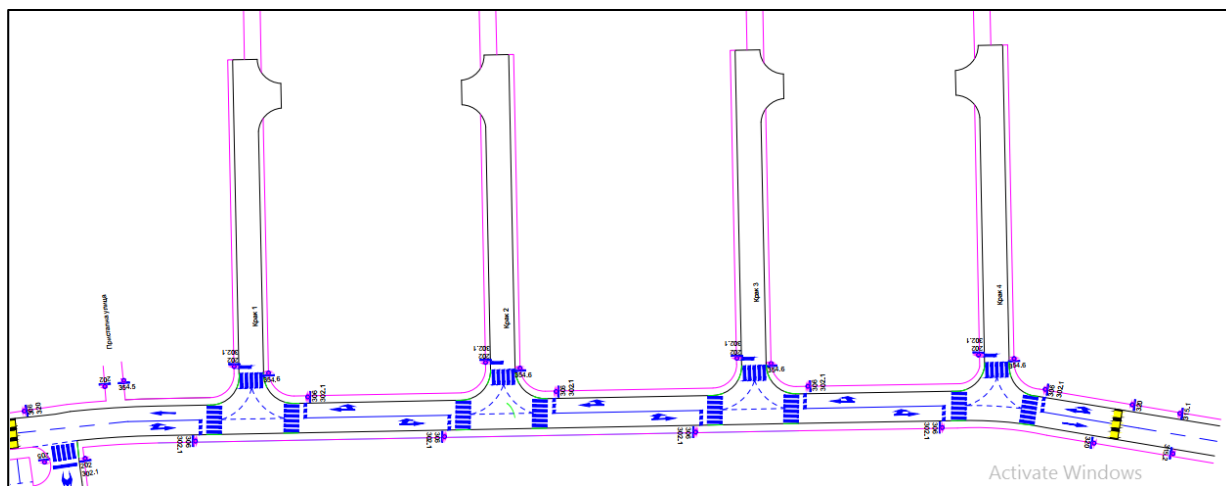
Слика 12-19: Графички прилози од проектна документација (ситуација, попречни профили, карактеристичен напречен пресек и детали, сообраќајно решение) за изградба на дел од улица Орце Николов во локалитет Шумски расадник
