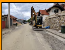
Изградба на атмосферска канализација во населба Милково Брдо 2
